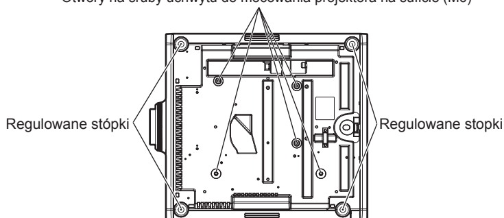
Położenie gwintowanych otworów do montażu uchwytu do mocowania na suficie oraz regulowanych stópek.
